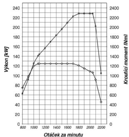
IVECO F2BE 1682G (EURO 3)
